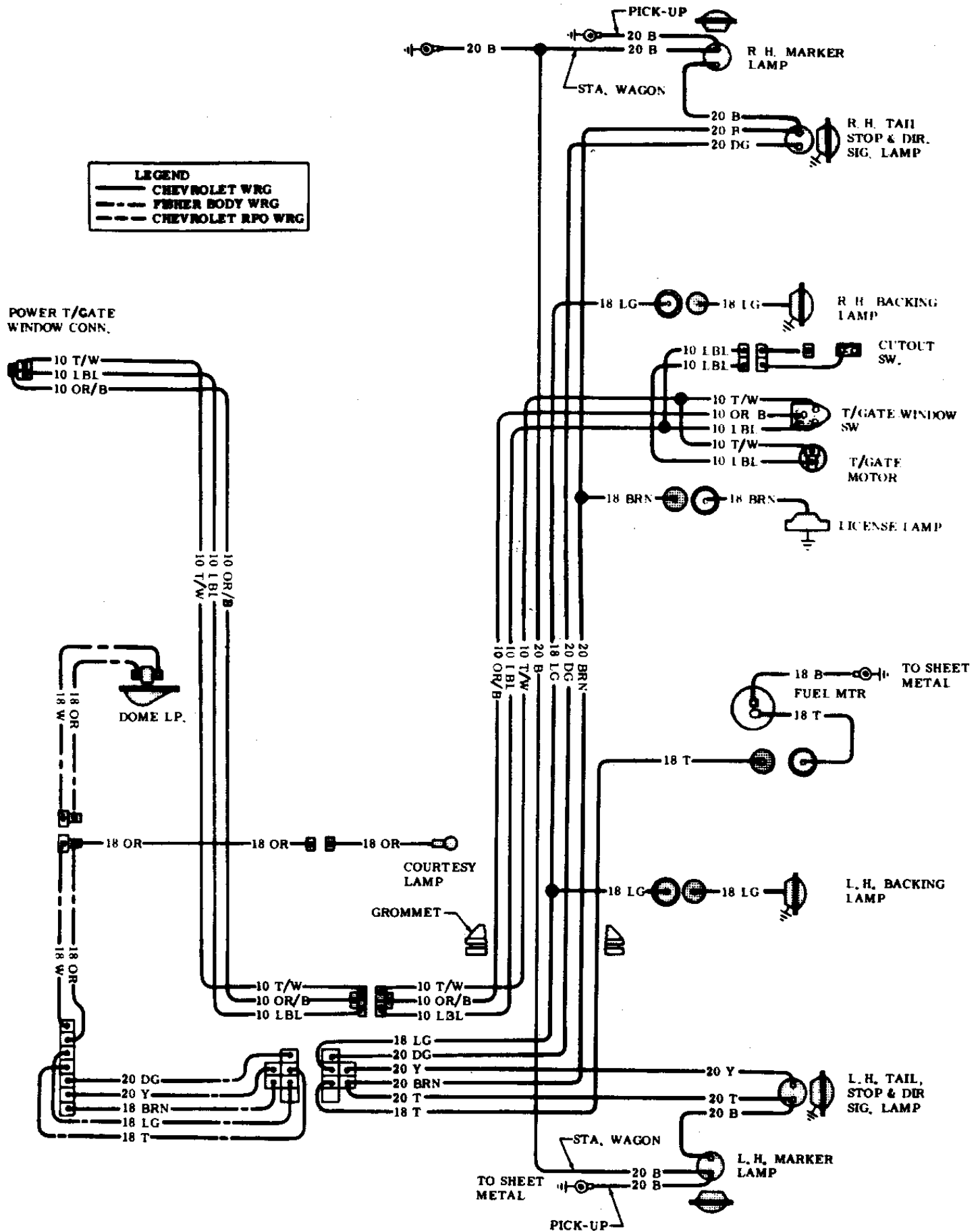
1970-72 Chevelle Wagon & El Camino Body & Rear Lights
