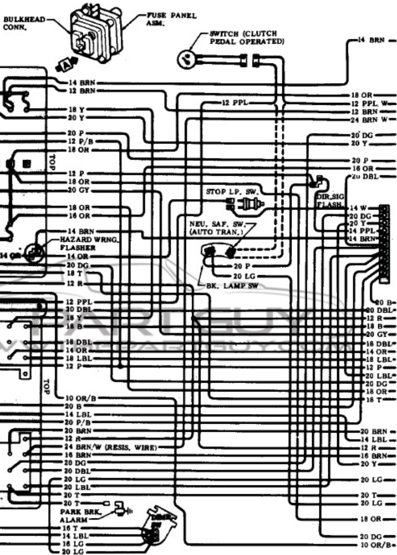
1969 Chevelle & El Camino Fuse Panel
