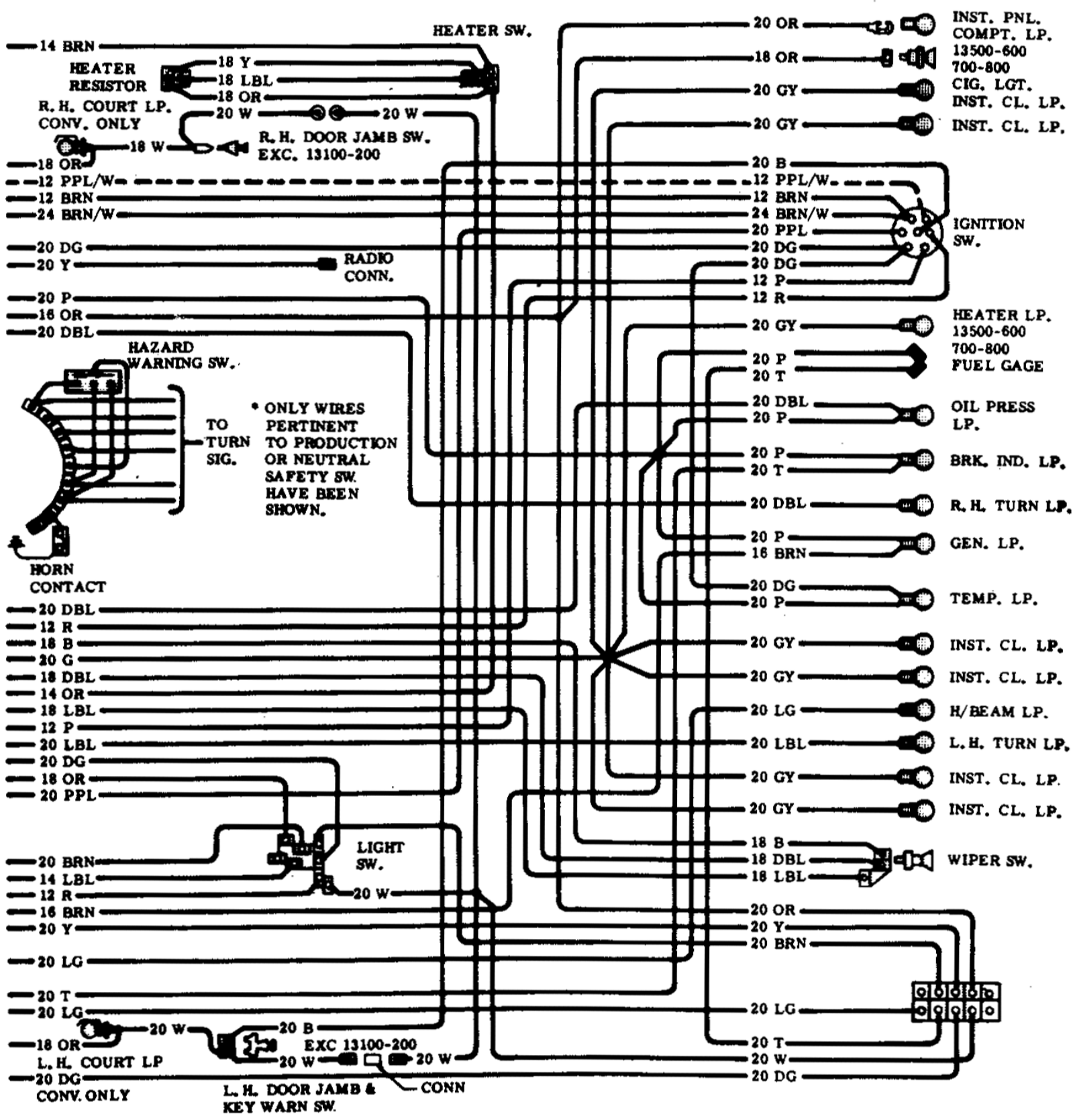
1968 Chevelle & El Camino Instrument Panel & Cluster
