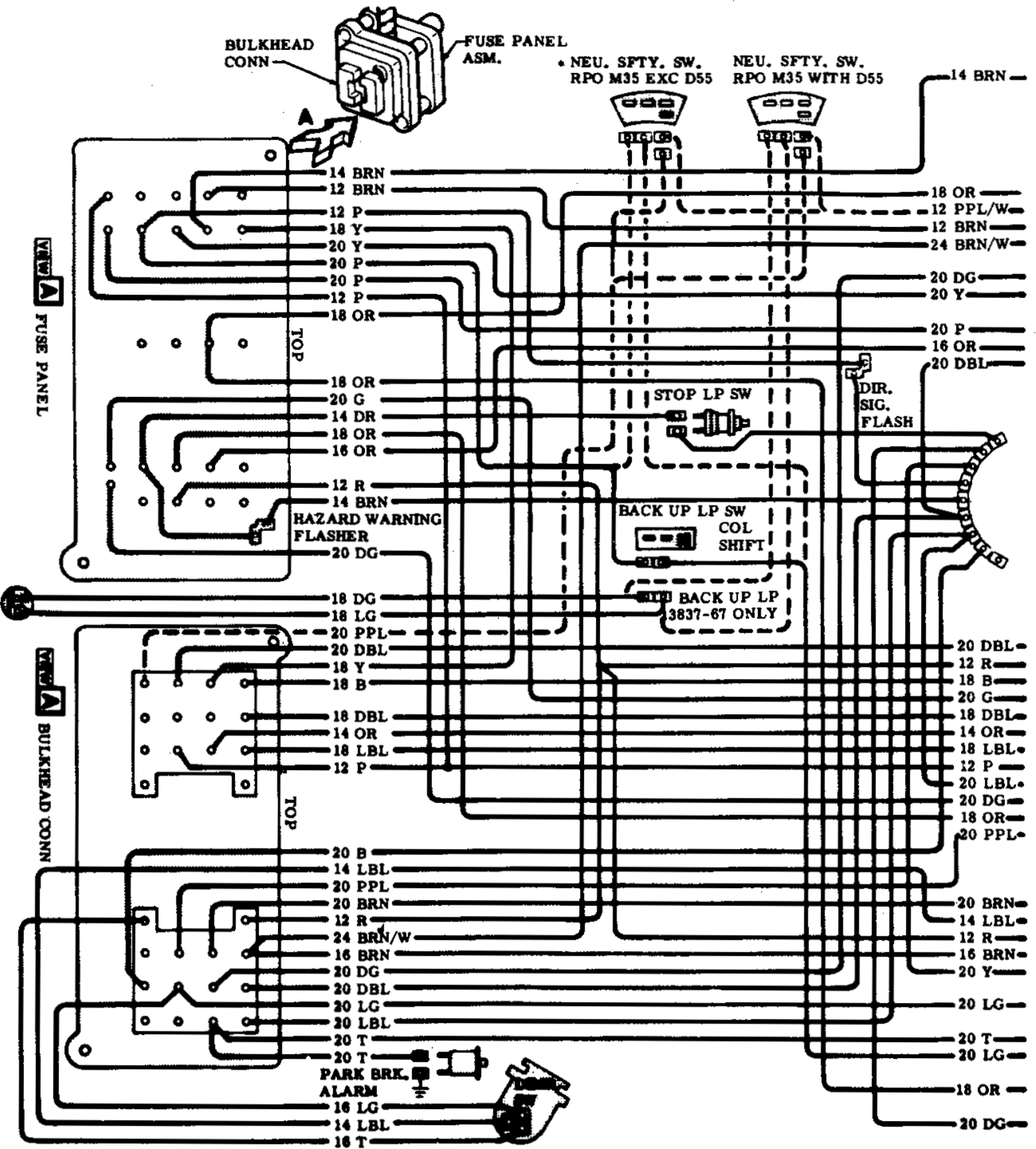
1968 Chevelle & El Camino Fuse Panel
