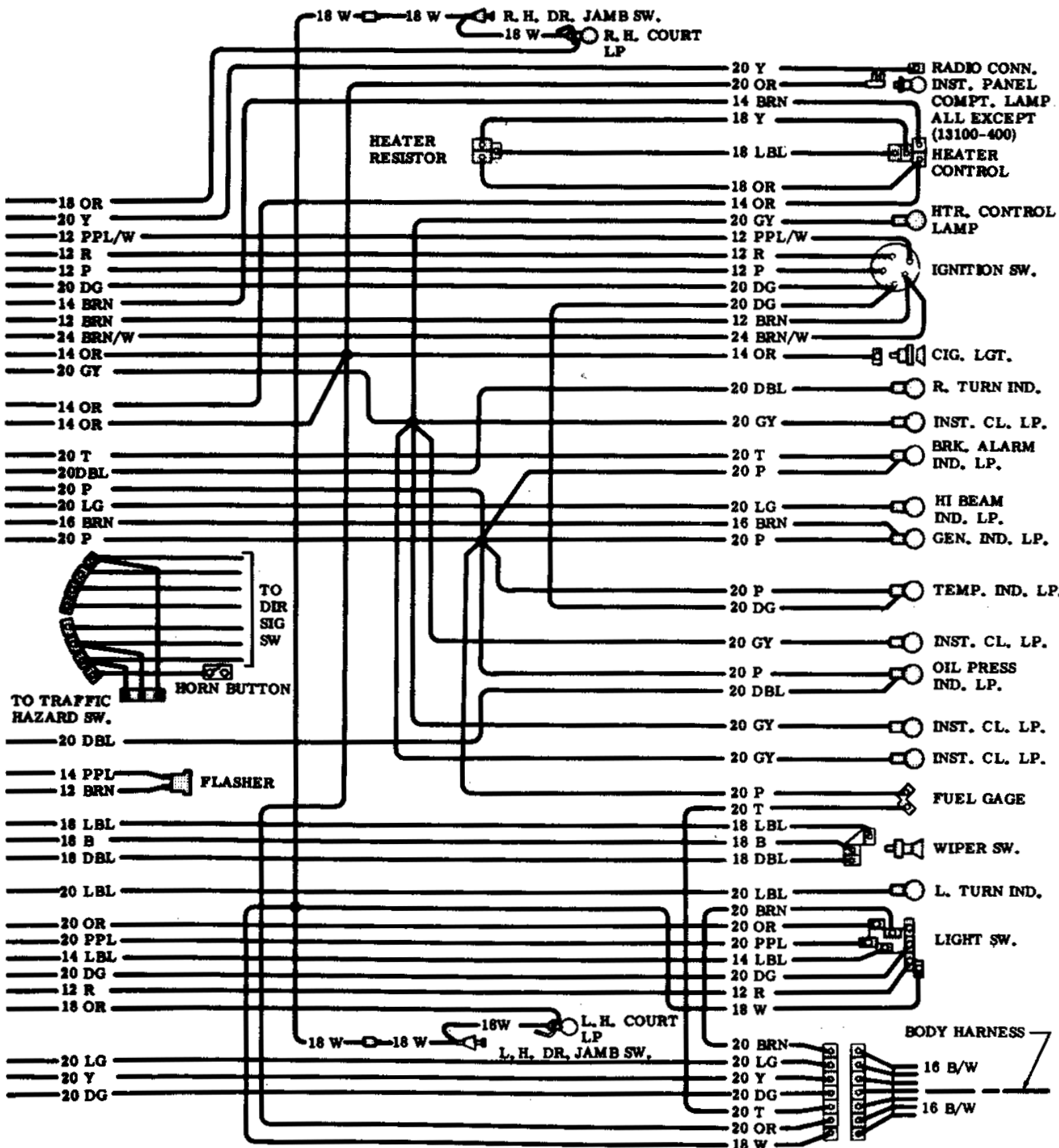
1967 Chevelle & El Camino Instrument Panel & Cluster
