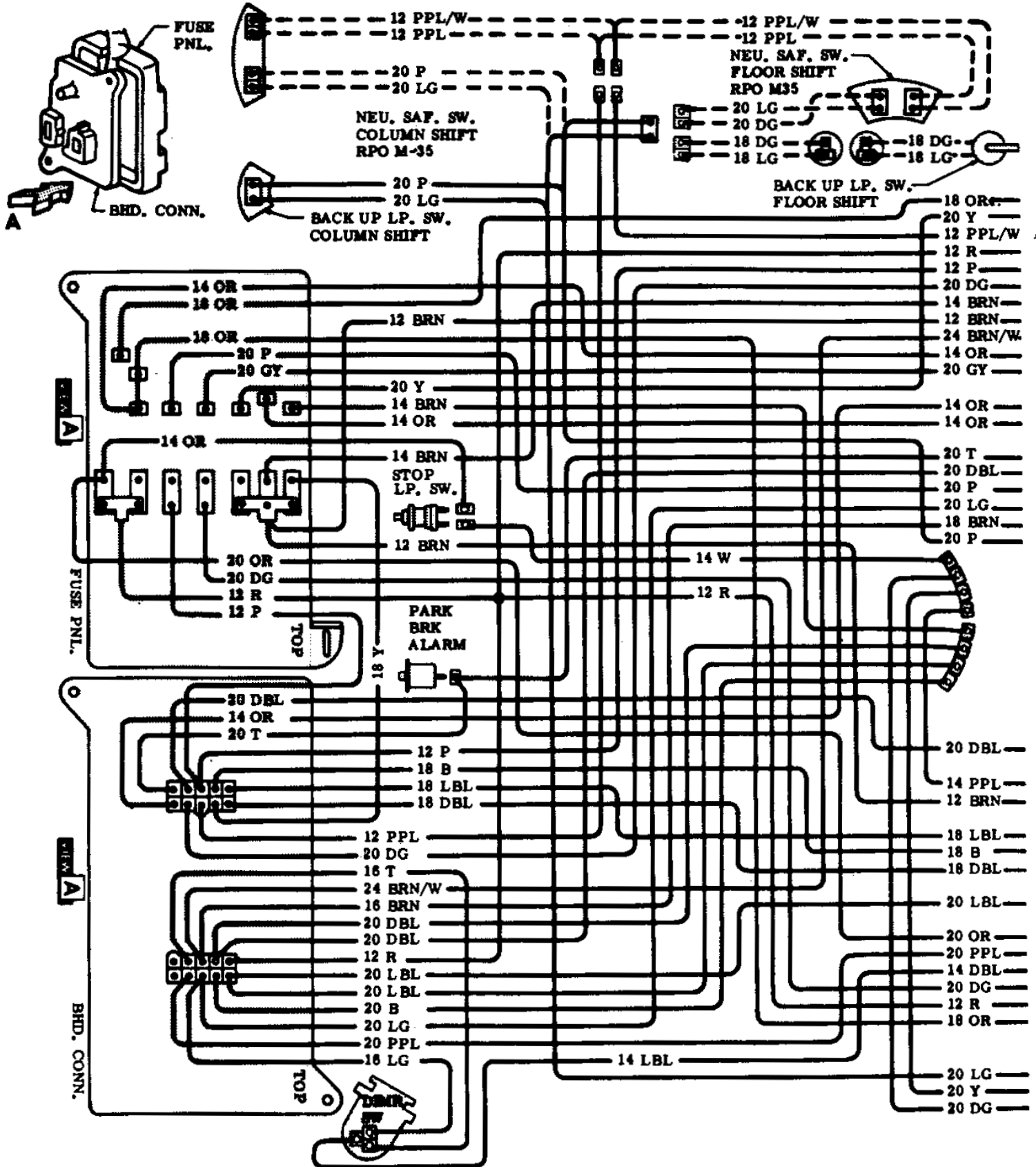
1967 Chevelle & El Camino Fuse Panel
