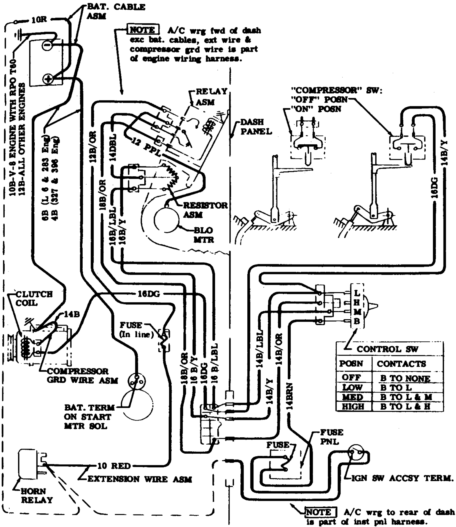
1967 Chevelle & El Camino A/C & Heater Wiring Diagram
